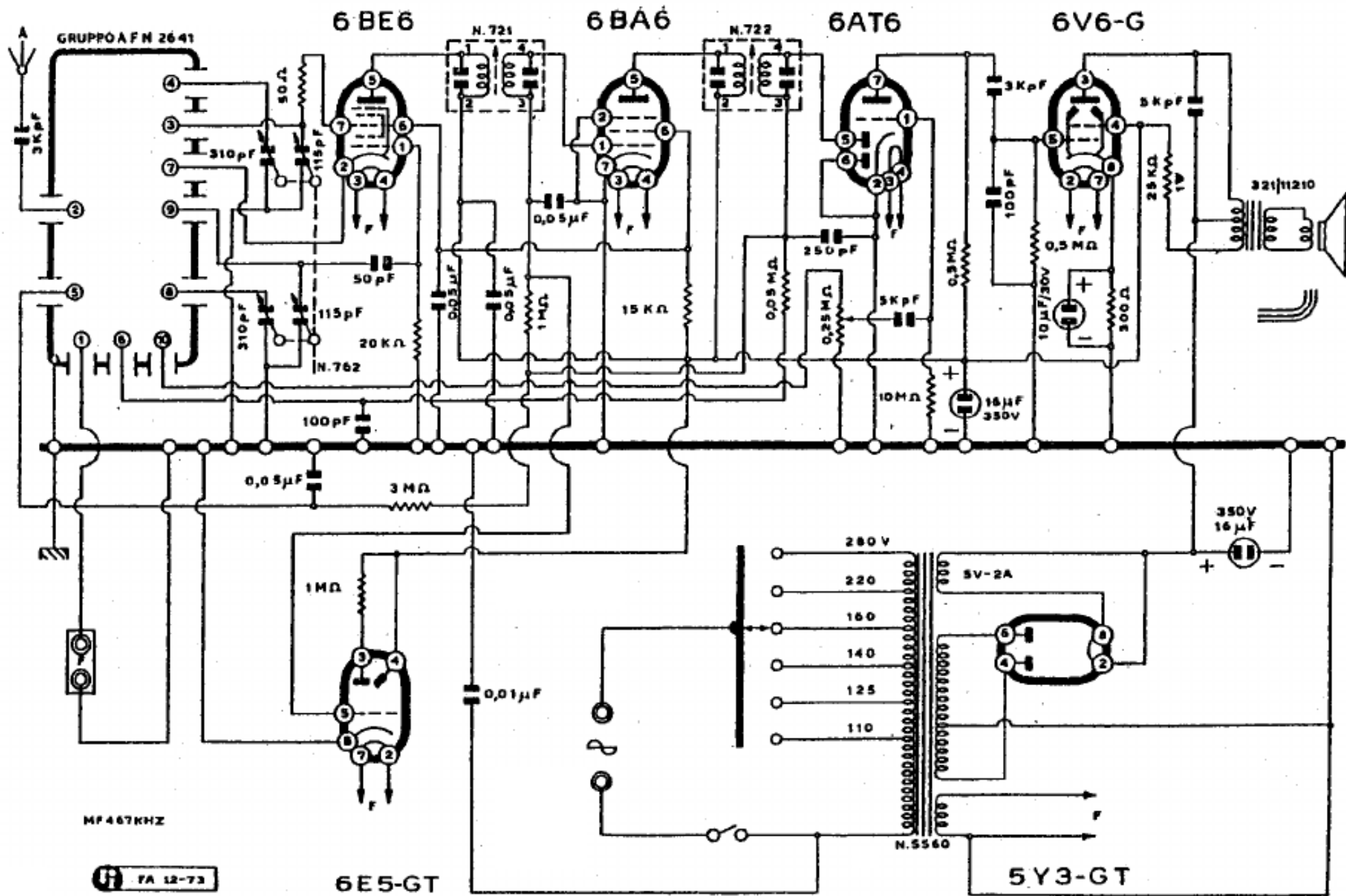
GELOSO S.A. - Modd. Super G 118 - G 119 - G 120
